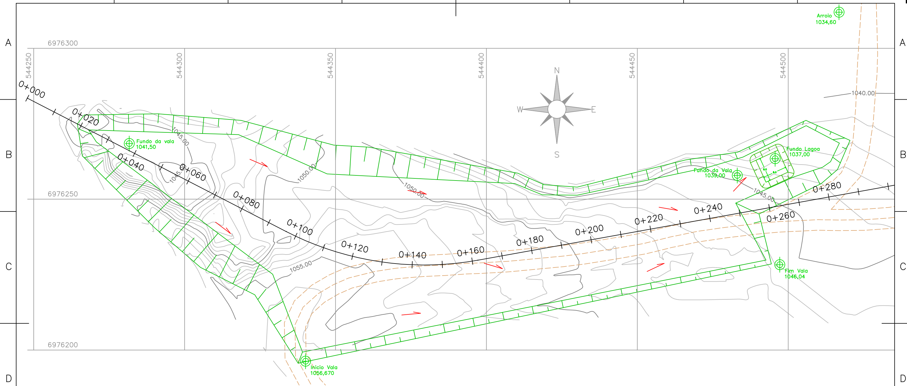
Planialtimétrico e Projeto da Vala Escala 1:750
